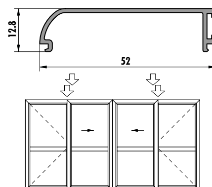
9284 (0,257 kg/m)
