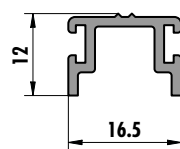
6287 (0,173 kg/m)
