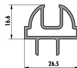
6266 (0,383 kg/m)
