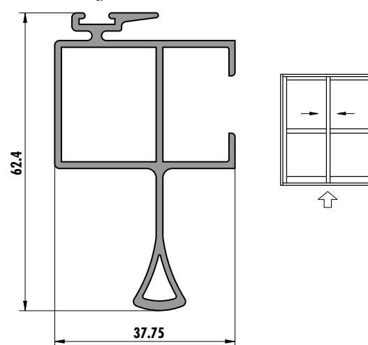
6208 (0,813 kg/m)
