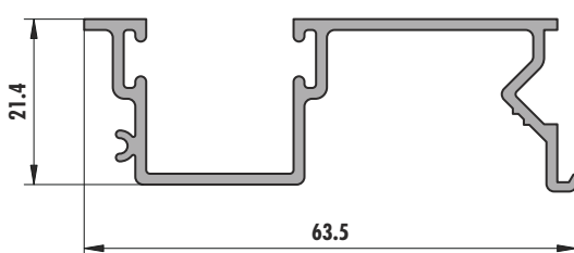
6243 (0,548 kg/m)
