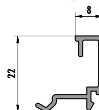
6238 (0,189 kg/m)
