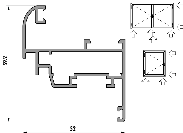
6234 (0,888 kg/m)
