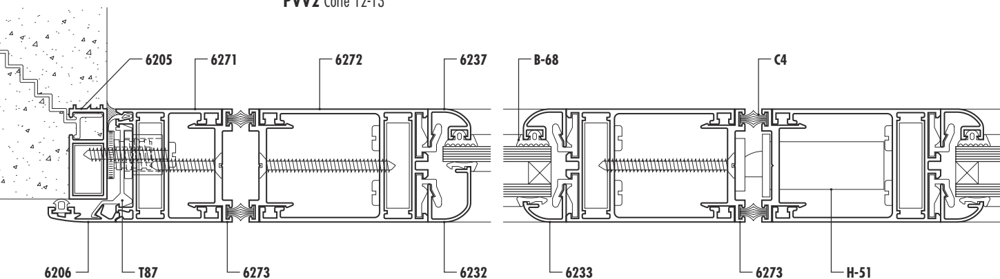
PVV2 Corte 12-13
