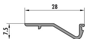
6299 (0,119 Kg/m)
