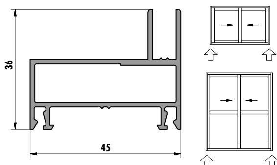
6201 (0,675 kg/m)
