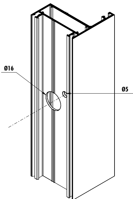
Mecanizado para T88
