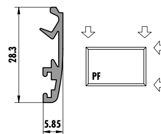
6206 (0,181 kg/m)
