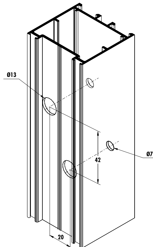
Mecanizado de marco para escuadra
