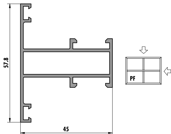
6221 (0,767 kg/m)
