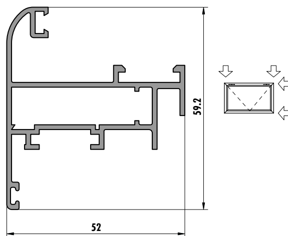
6236 (0,902 kg/m)
