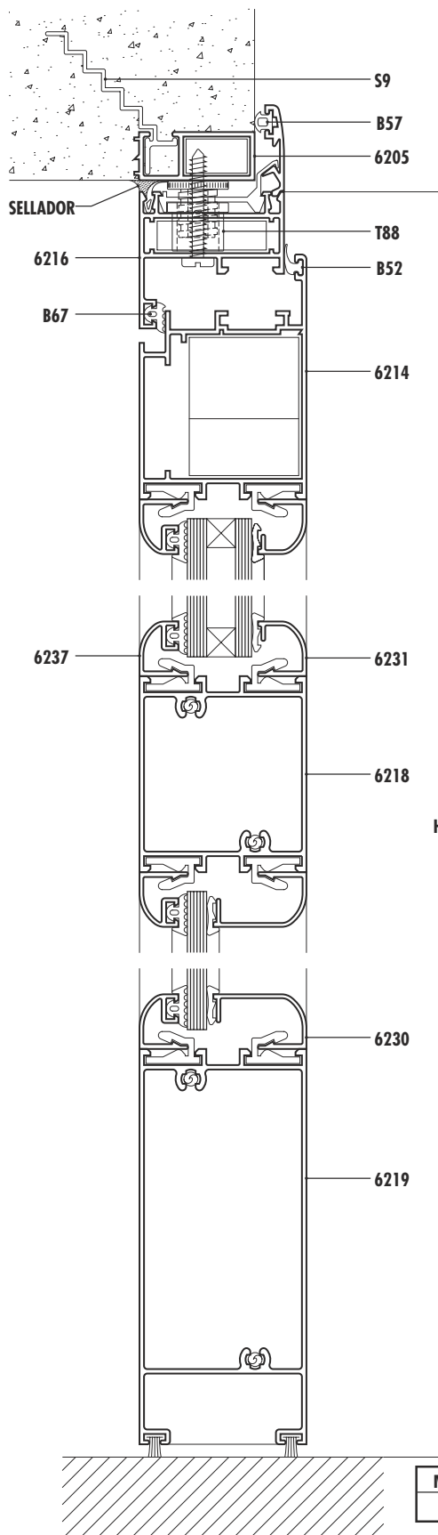
PRC Corte 1-2-3
