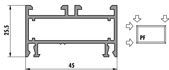
6269 (0,670 kg/m)
