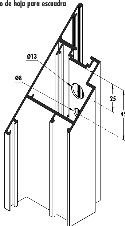
Mecanizado de hoja para escuadra
