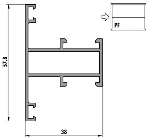
6264 (0,719 kg/m)
