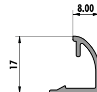
6233 (0,146 kg/m)
