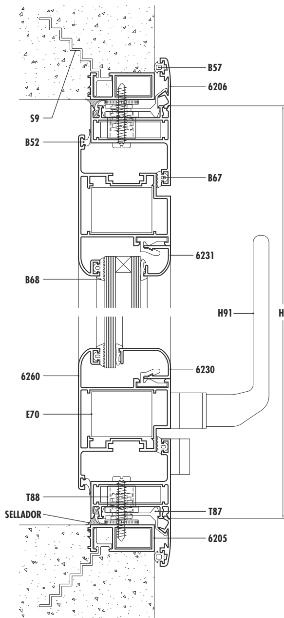
VPC Corte 5-6
