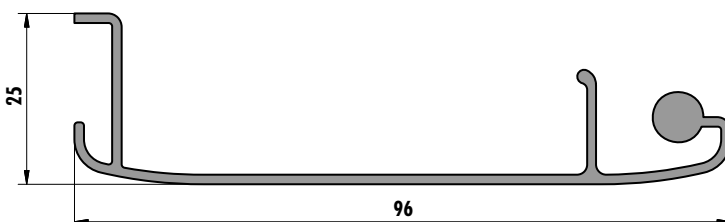
6245 (0,678 kg/m)
