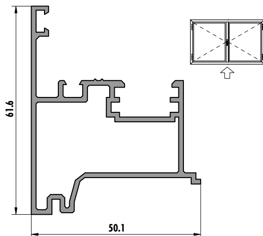
6223 (0,921 kg/m)
