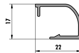
6232 (0,194 kg/m)
