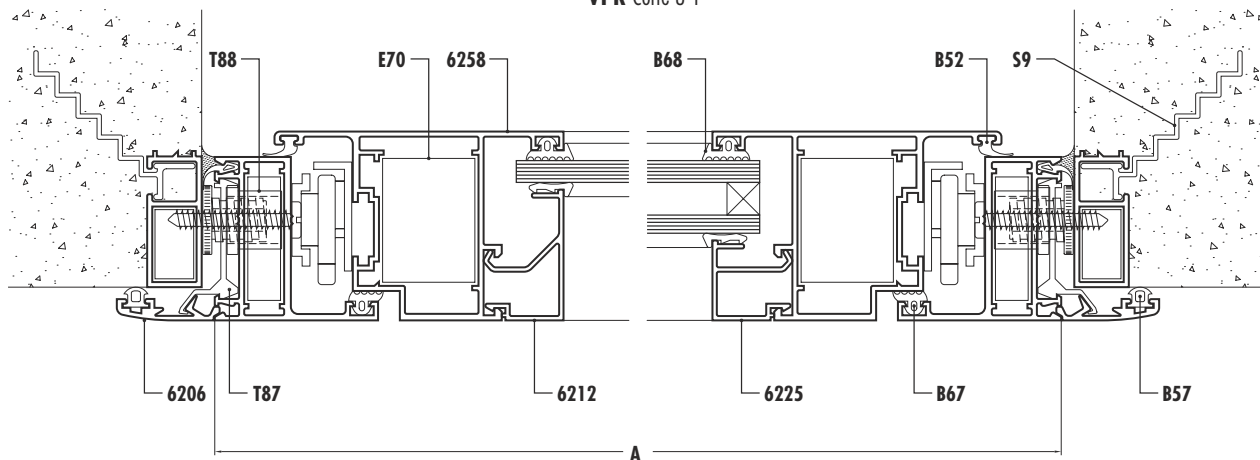
VPR Corte 3-4
