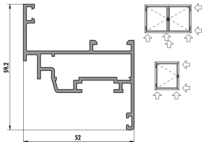
6211 (0,848 kg/m)
