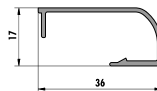
6257 (0,240 kg/m)
