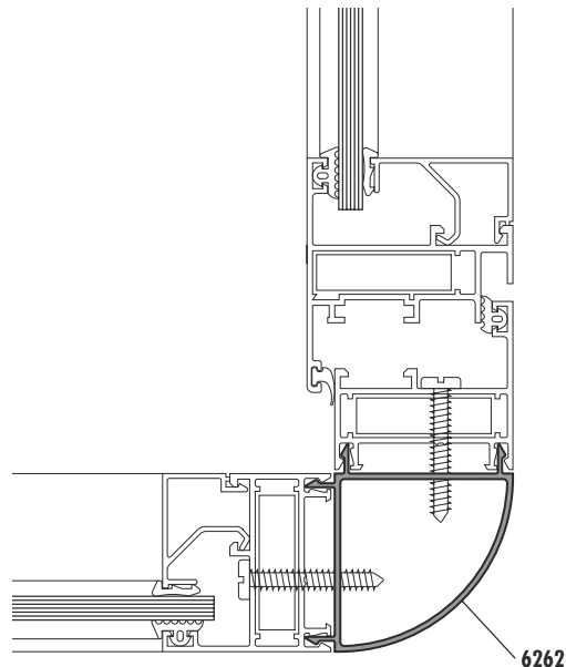
Perfil de acople a 90° Corte 6
