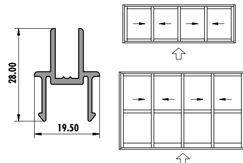
6246 (0,291 kg/m)
