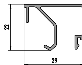
6217 (0,294 kg/m)
