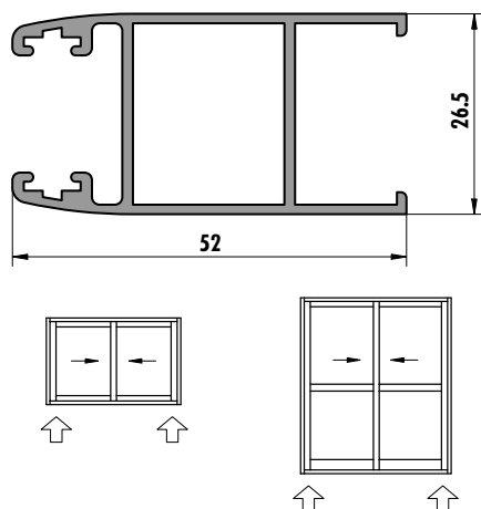
6248 (0,635 kg/m)
