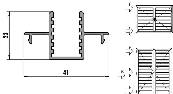
6280 (0,367 kg/m)
