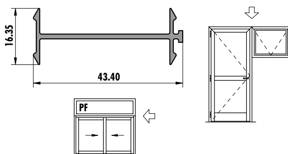
6213 (0,257 kg/m)
