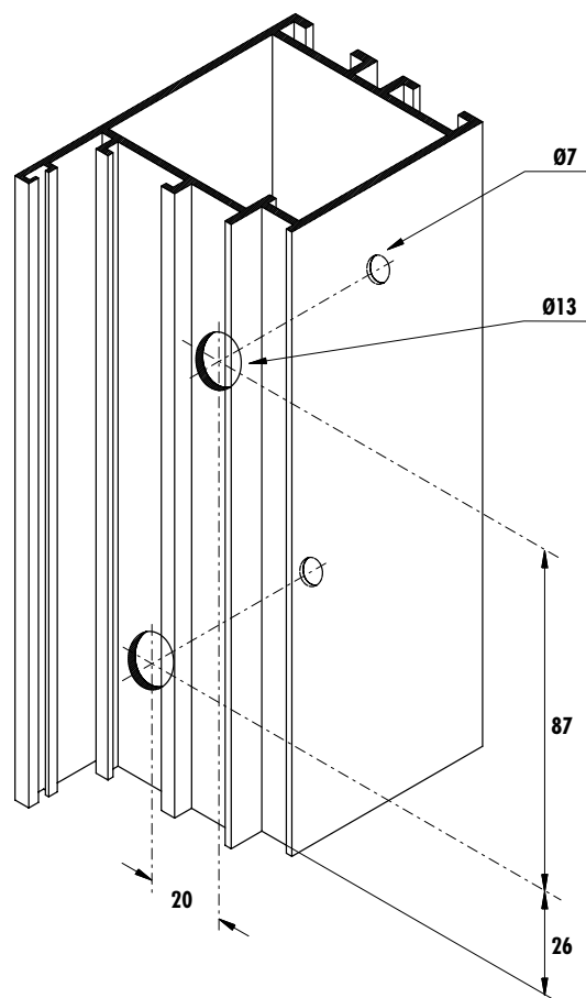
Mecanizado para zócalo
