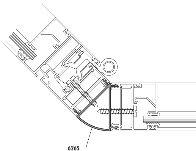
Perfil de acople a 135° Corte 1
