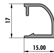
6231 (0,170 kg/m)
