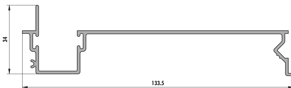
6244 (0,913 kg/m)
