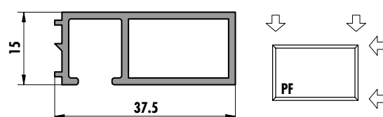
6205 (0,397 kg/m)
