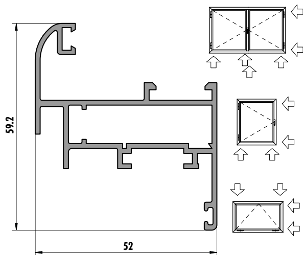
6235 (0,902 kg/m)
