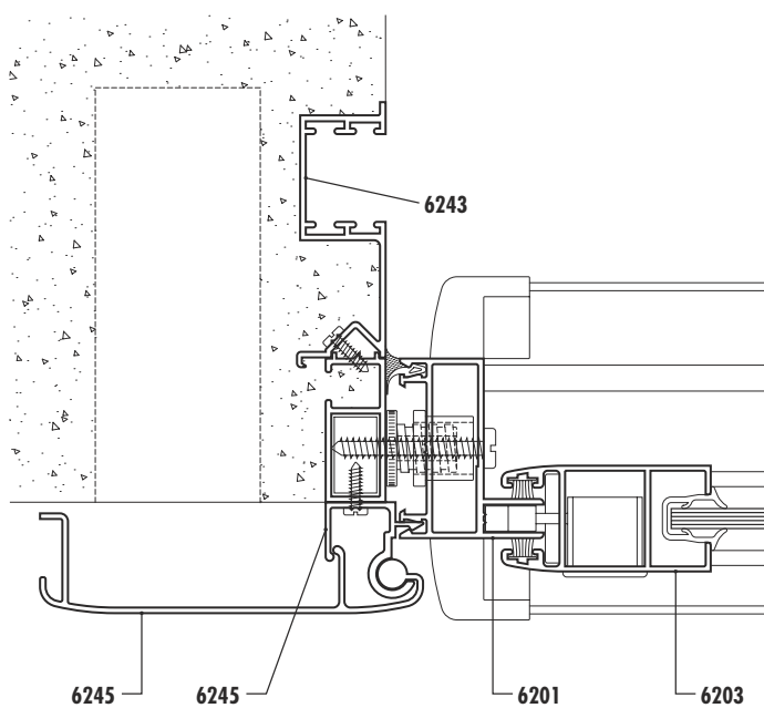
Detalle guía común
