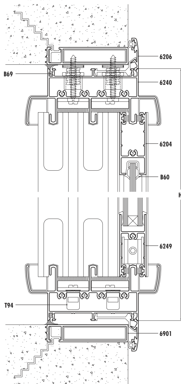
VPC3H Corte 9-10
