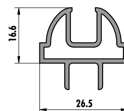
6267 (0,383 kg/m)
