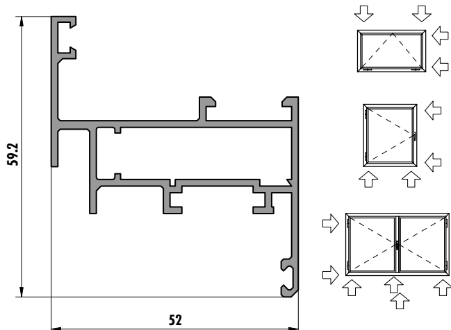
6215 (0,864 kg/m)
