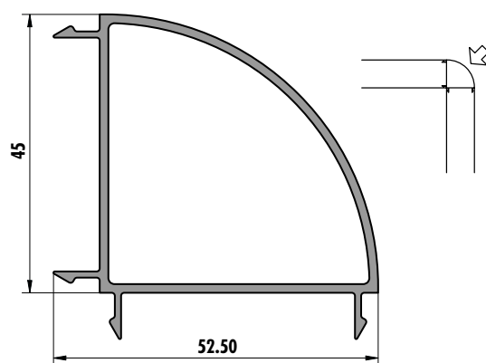
6262 (0,680 kg/m)
