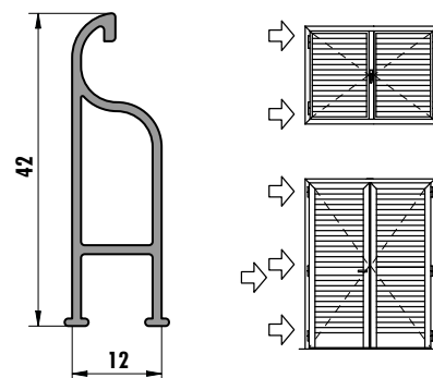
6278 (0,319 kg/m)
