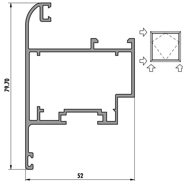
6260 (1,099 kg/m)
