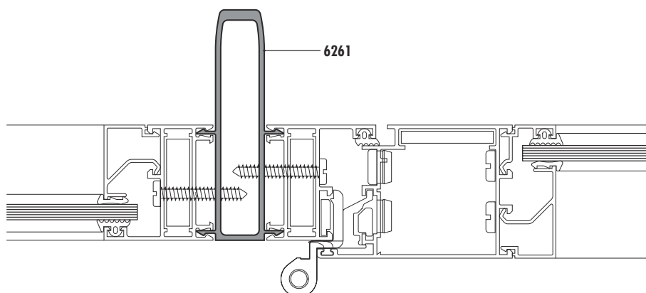
Columna de acople reforzado Corte 2
