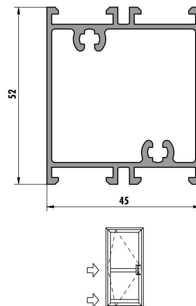
6274 (1,029 kg/m)
