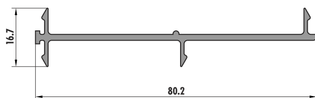
4148 (0,346 Kg/m)
