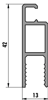
6255 (0,424 kg/m)
