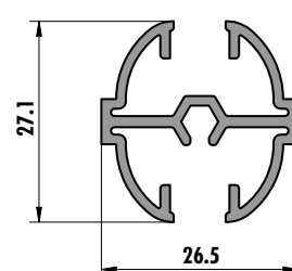
6268 (0,429 kg/m)
