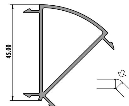
6265 (0,543 kg/m)
