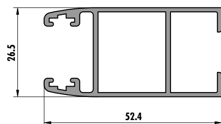
6203 (0,664 kg/m)
