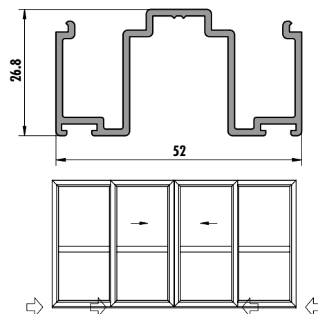
6282 (0,605 kg/m)
