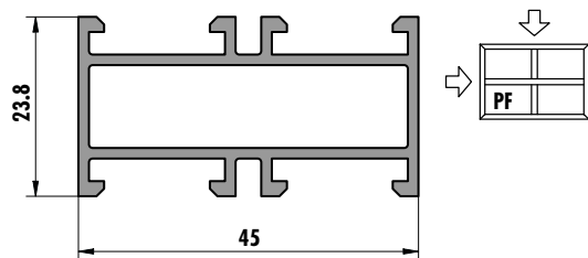
6270 (0,651 kg/m)
