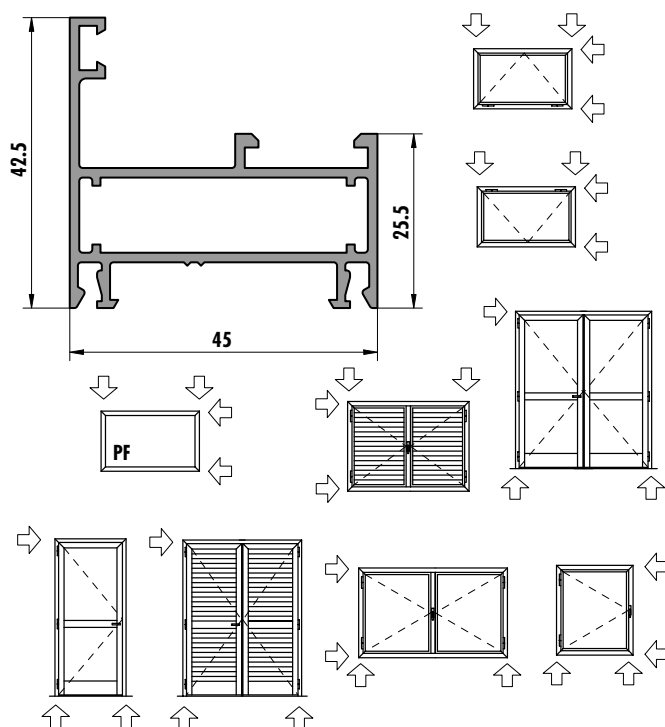
6216 (0,726 kg/m)
