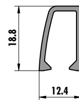
6228 (0,186 kg/m)
