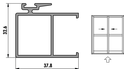
6250 (0,583 kg/m)
