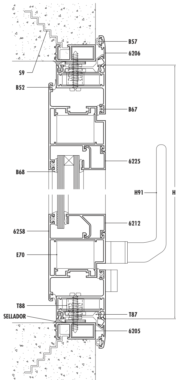
VPR Corte 1-2
