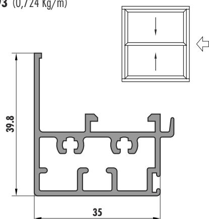
6293 (0,724 Kg/m)
