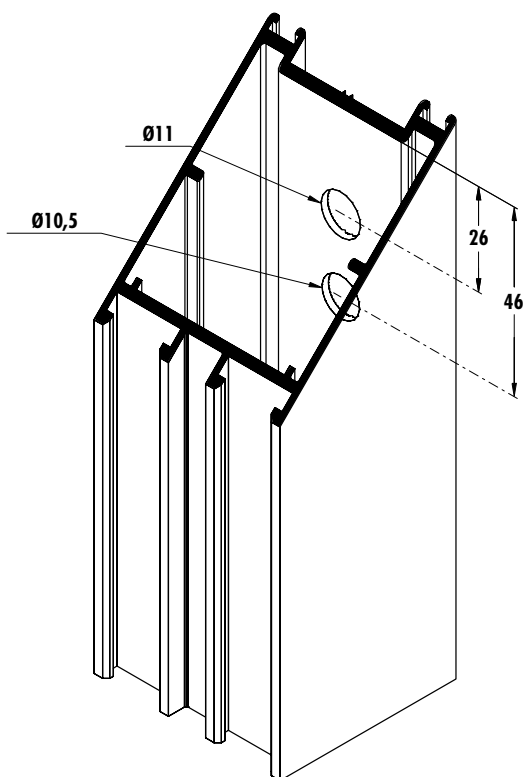
Mecanizado de hoja para escuadra
