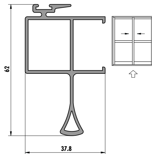
6251 (0,783 kg/m)
