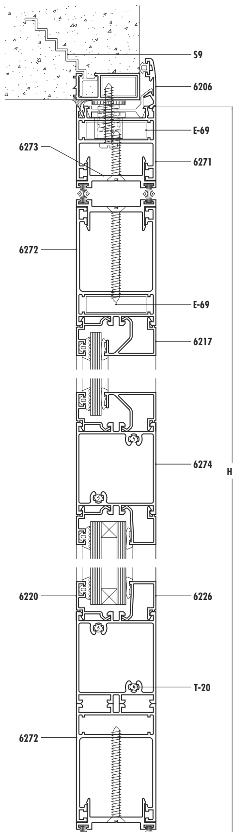
PVVR Corte 1-2-3
