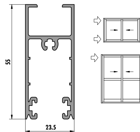
6204 (0,705 kg/m)
