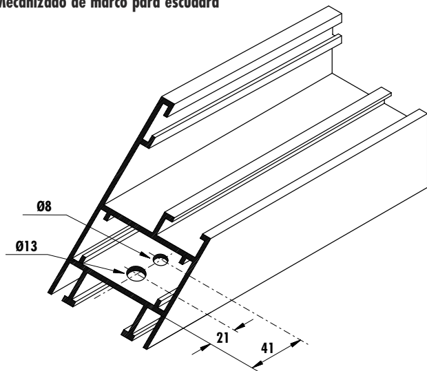
Mecanizado de marco para escuadra
