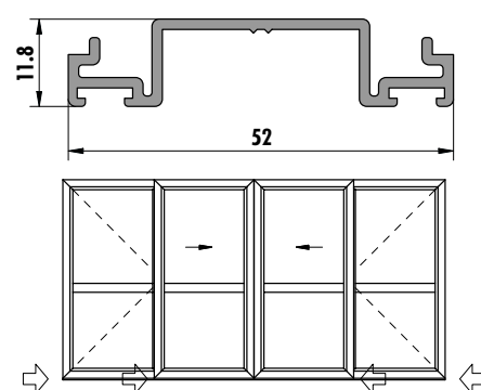
6283 (0,381 kg/m)
