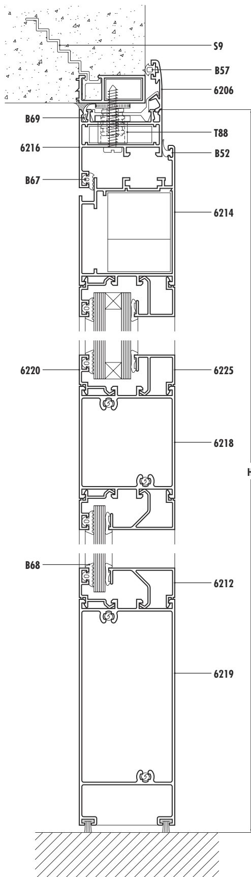
PRR Corte 1-2-3
