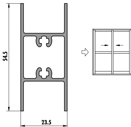
6253 (0,689 kg/m)
