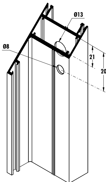
Mecanizado de marcos para escuadra
