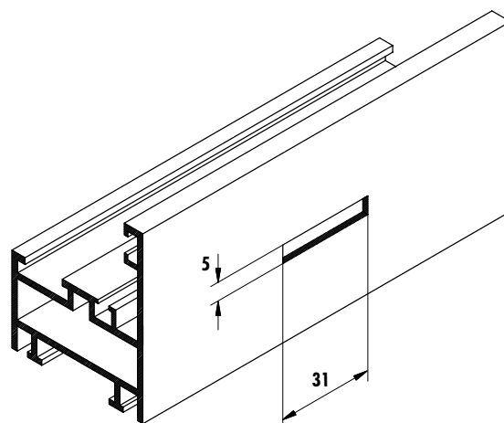
Mecanizado para drenaje
