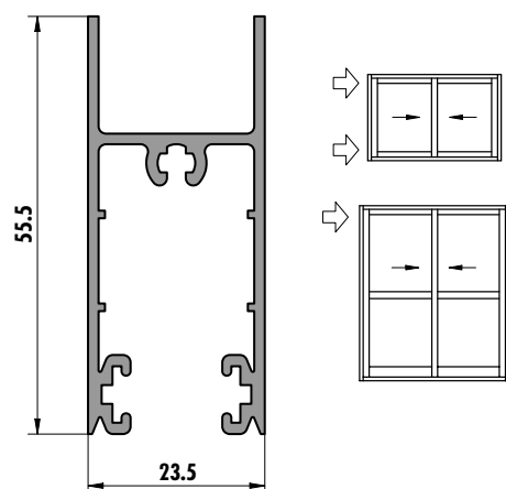
6249 (0,675 kg/m)
