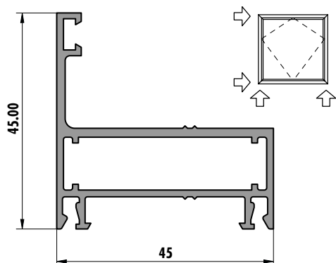
6259 (0,726 kg/m)
