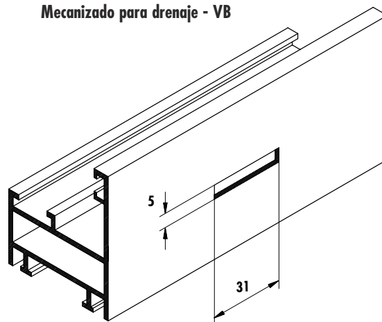
Mecanizado para drenaje - VB
