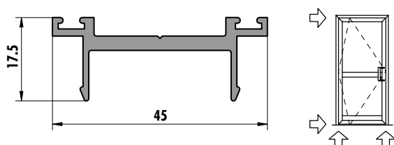
6273 (0,456 kg/m)
