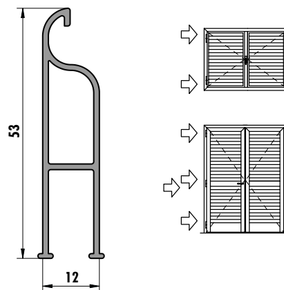
6279 (0,392 kg/m)
