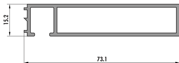
6902 (0,470 Kg/m)
