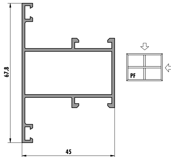
6222 (0,842 kg/m)
