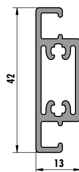
6256 (0,508 kg/m)
