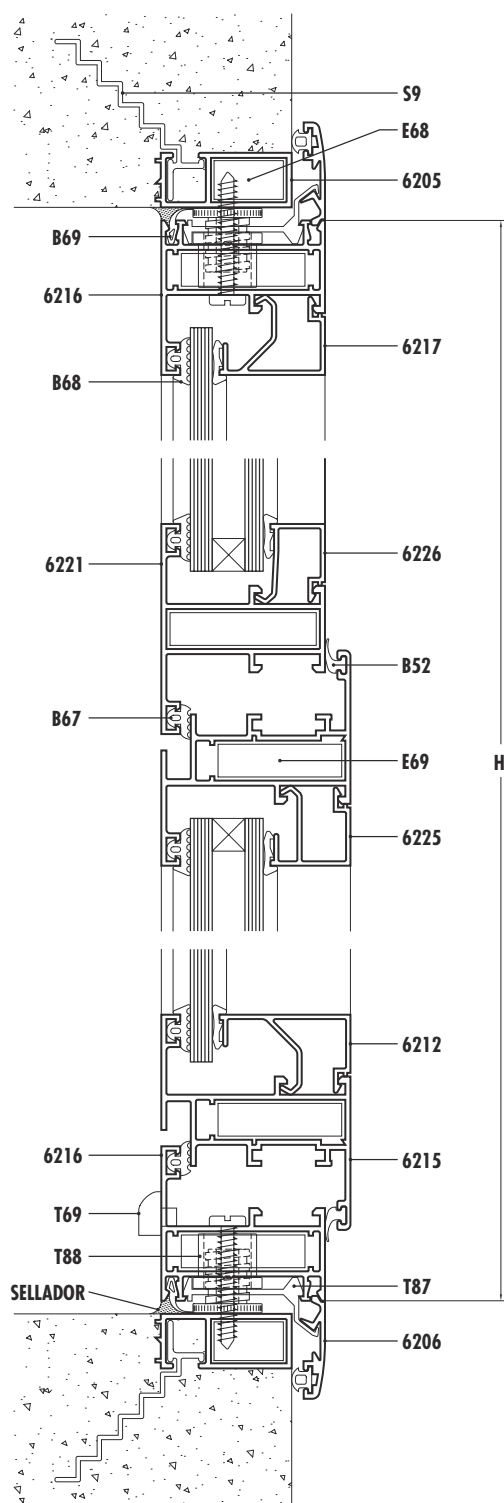
VADCR / PF Corte 1-2-3
