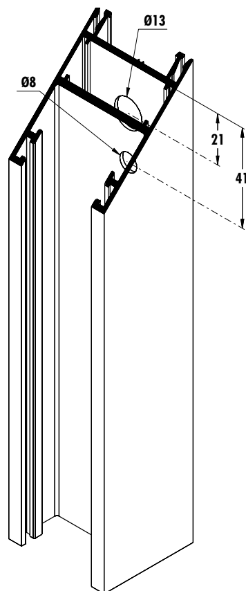
Mecanizados escuadra hoja
