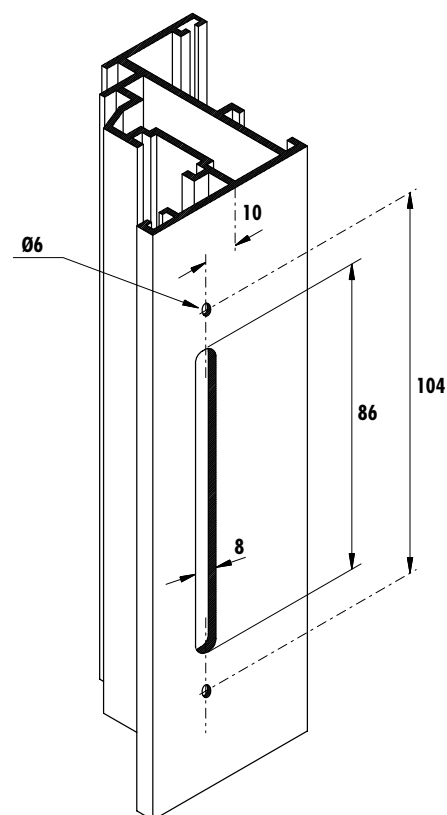
Mecanizado para H48
