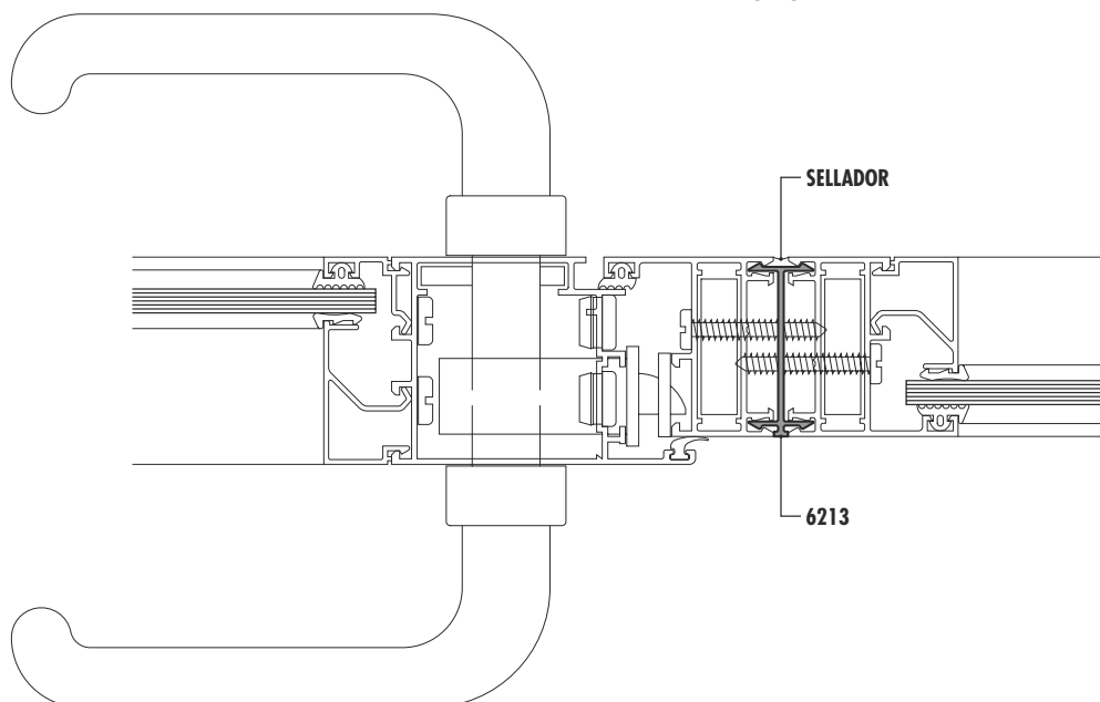
Perfil de acople plano Corte 3
