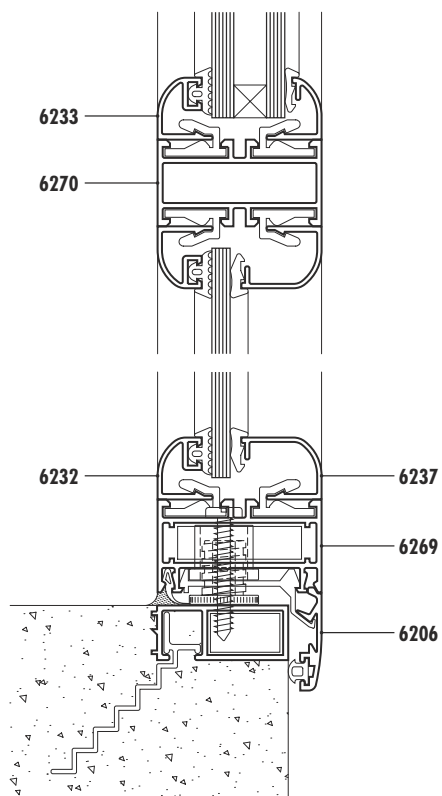
Detalle zócalo bajo
