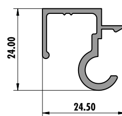
6254 (0,302 kg/m)
