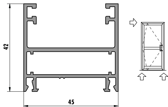
6271 (0,880 kg/m)
