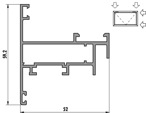
6227 (0,864 kg/m)
