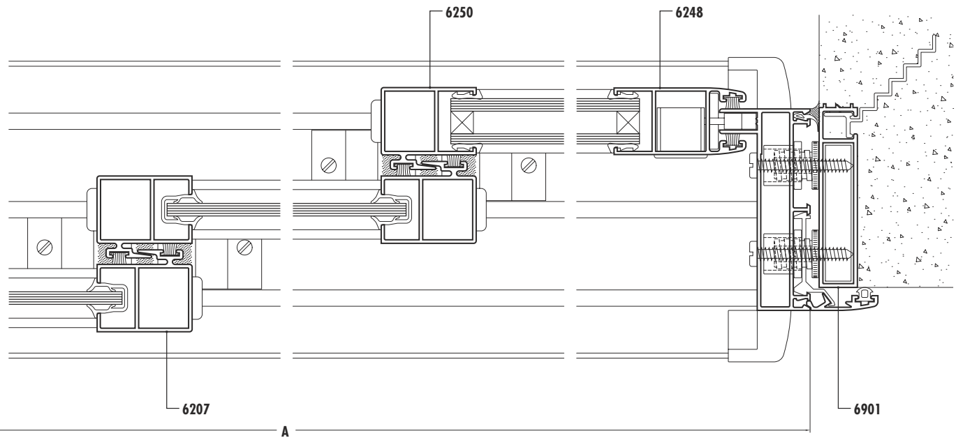
VPCVR Corte 15-16
