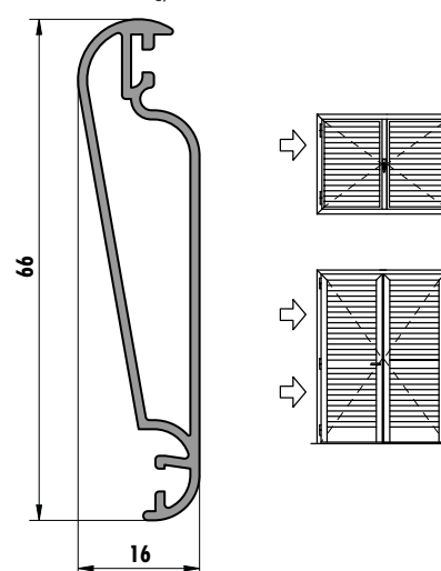
6277 (0,518 kg/m)
