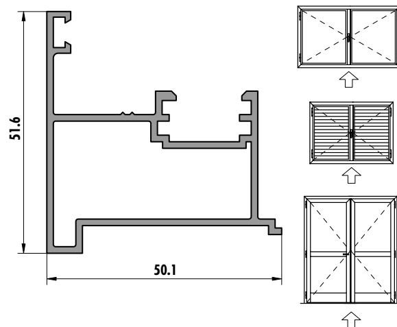
6224 (0,794 kg/m)
