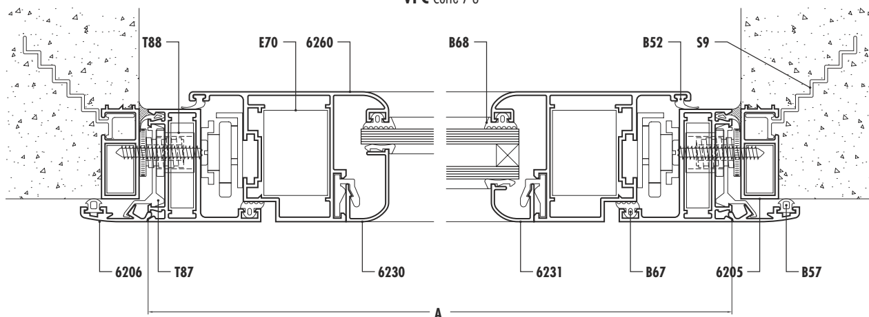
VPC Corte 7-8
