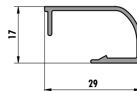
6230 (0,213 kg/m)
