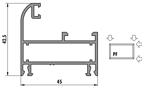
6229 (0,764 kg/m)
