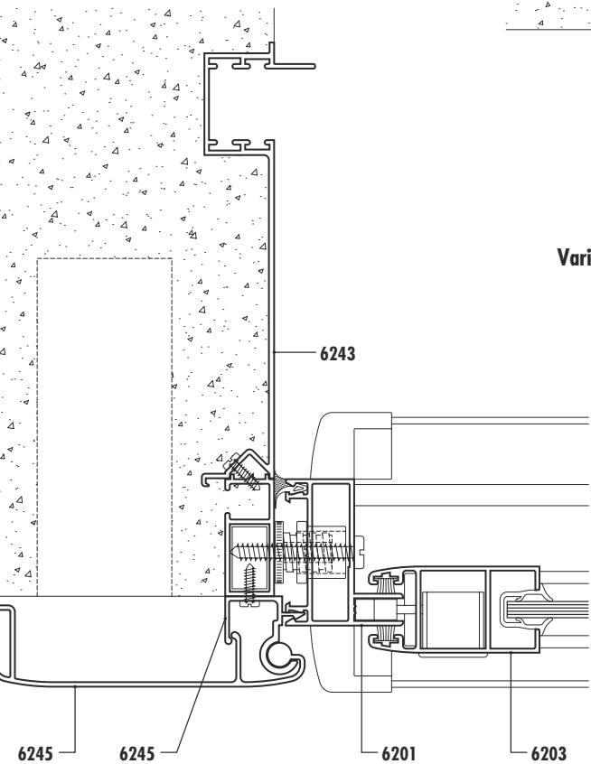
Detalle guía barrio
