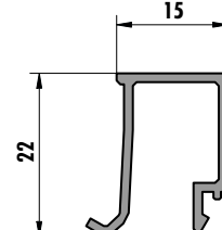
6226 (0,211 kg/m)
