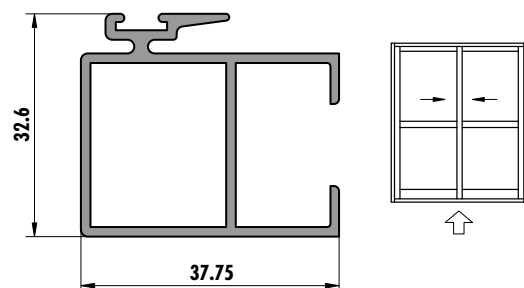
6207 (0,613 kg/m)
