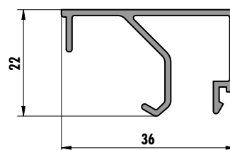
6212 (0,316 kg/m)
