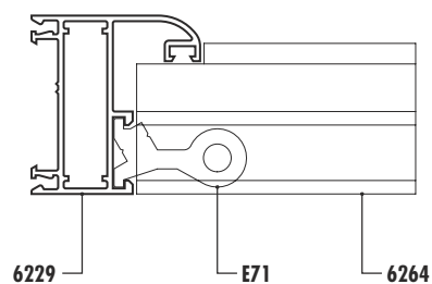
Detalle ensamble con travesaño
