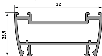
6286 (0,740 kg/m)
