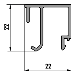
6225 (0,257 kg/m)
