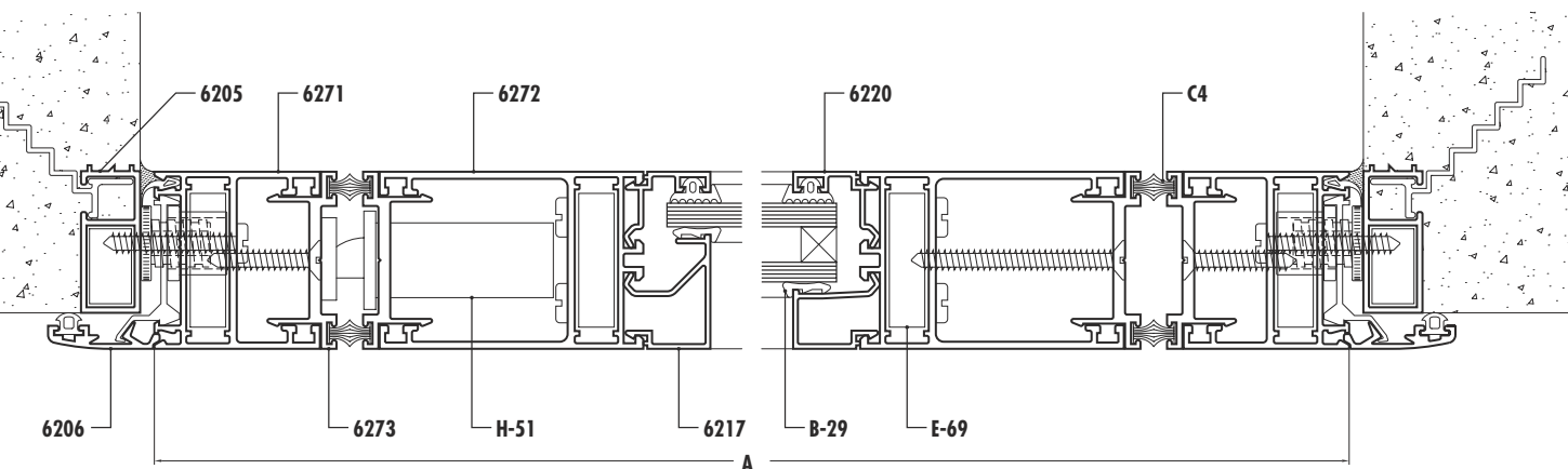
PVVR Corte 4-5
