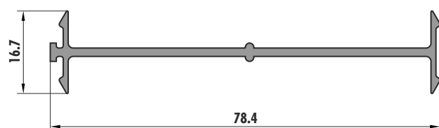
6903 (0,462 Kg/m)
