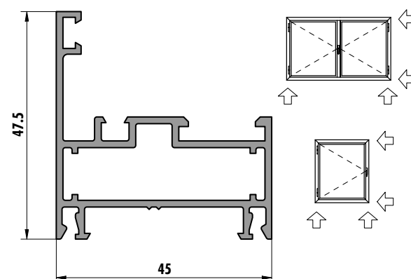
6210 (0,789 kg/m)
