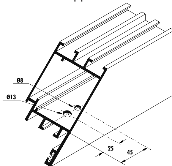
Mecanizado de hoja para escuadra
