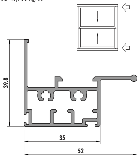
6295 (0,783 Kg/m)
