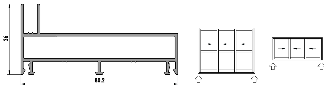
6241 (0,975 kg/m)
