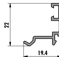
6220 (0,176 kg/m)
