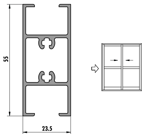
6239 (0,705 kg/m)
