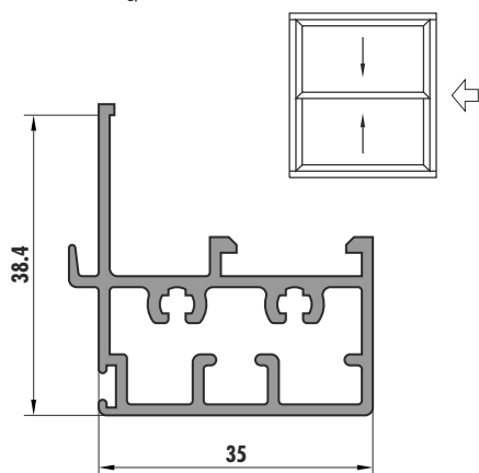
6294 (0,724 Kg/m)
