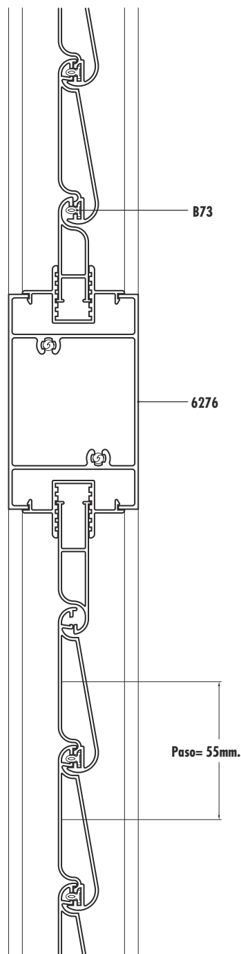
Detalle travesaño
