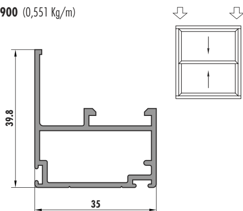
6901 (0,710 Kg/m)
