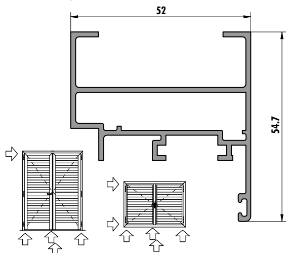
6275 (0,880 kg/m)
