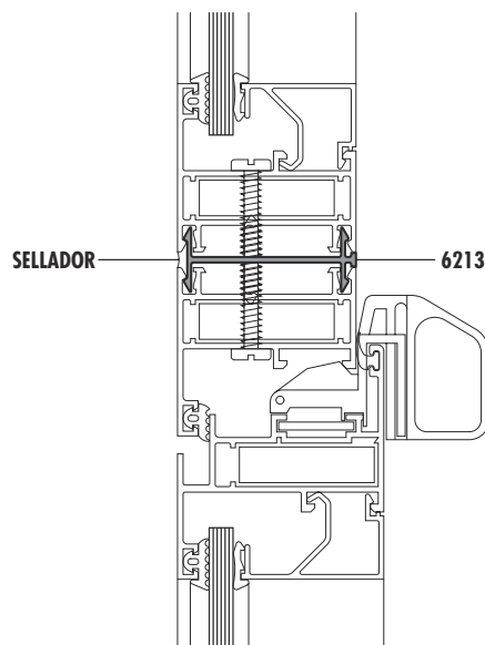
Perfil de acople a plano Corte 5
